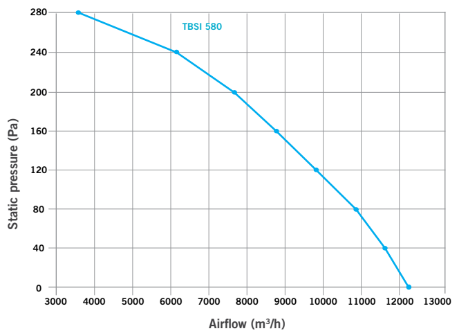
FAN CURVE
